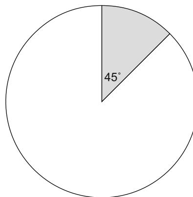
geheugengebruik
